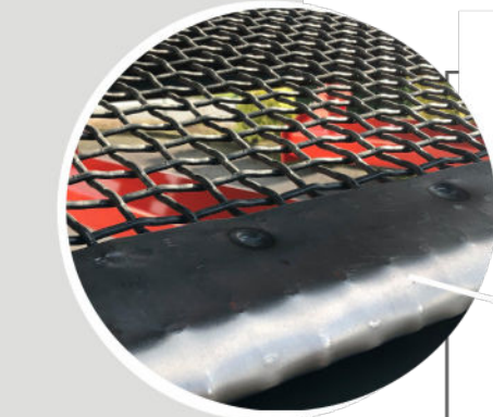
Crible vibrant : 2 fractions à un Tamis
