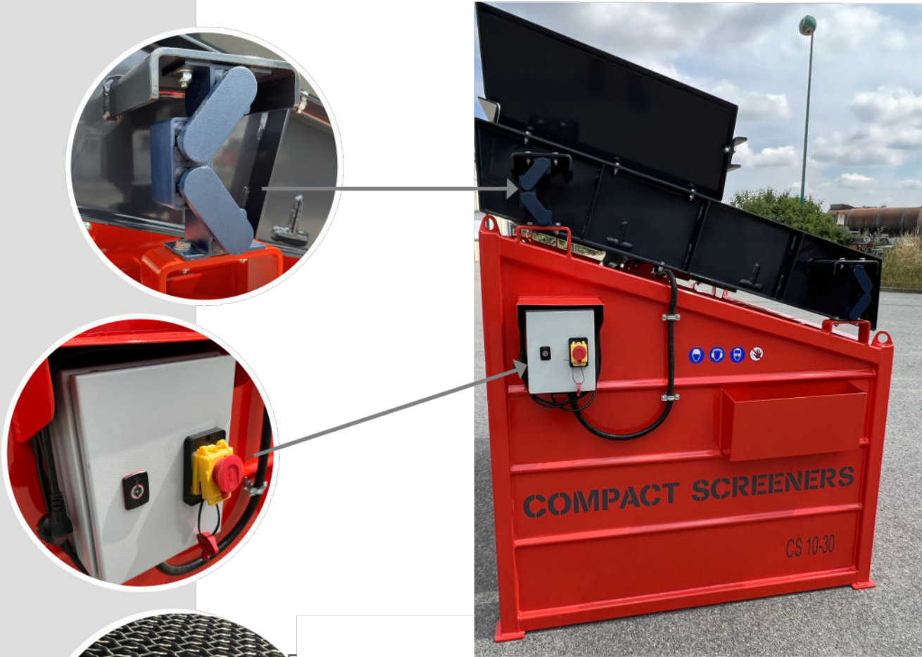
Crible vibrant : 2 fractions à un Tamis
